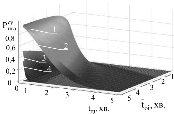
Рис. 2. Залежність показника якості \bar{t}_{оі} , хв. системи управління угруповання ППО ОСШР від математичного очікування часу отримання \bar{t}_{ді} , хв. розвідувальної інформації та часу \bar{t}_{ді} доведення цілевказівок
