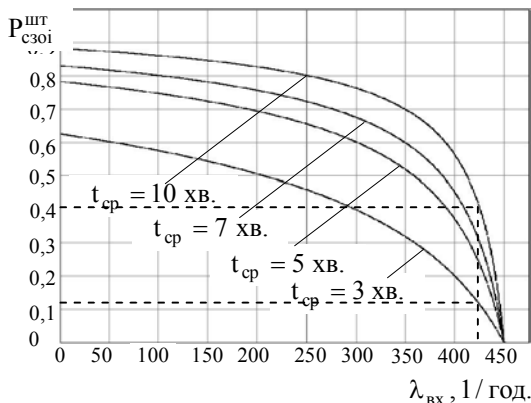
Рис. 1. Графіки залежності ймовірності своєчасності збору та обробки розвідувальних відомостей на СКП ППО і АА від інтенсивності вхідного потоку розвідувальних відомостей
