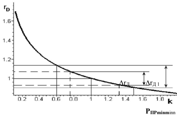
Рис. 2. Графічна залежність відносної дальності виявлення цілей від мінімального значення потужності сигналу
