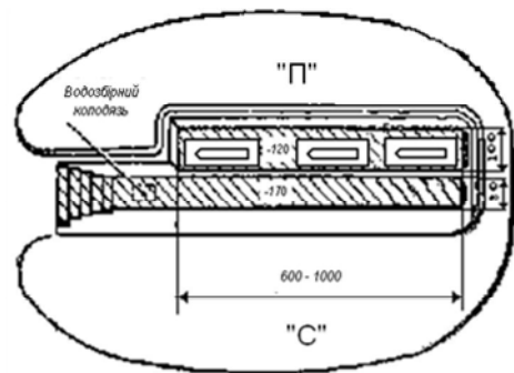
Рис. 5. Погрібець для боєприпасів (пропонуємий варіант)
