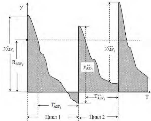
Рис. 2. Стохастична модель управління запасами авіаційних засобів ураження
