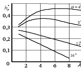
Рис. 11. Зависимость h_y^*(\lambda)
