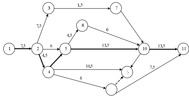
Рис. 1. Сіткова модель
