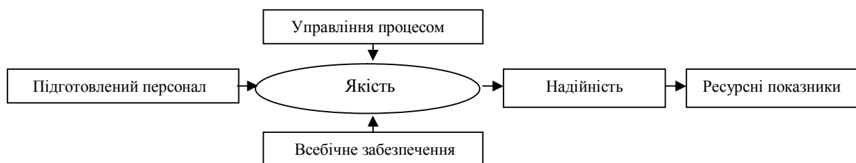
Рис. 3. Концептуальна схема
