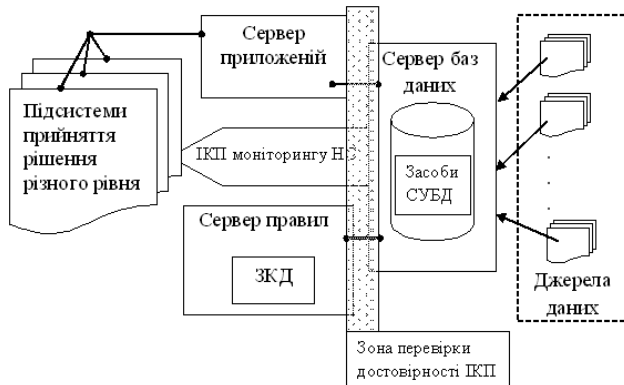
Рис. 5. Архітектура розміщення ЗКД для перевірки ІКП моніторингу НС в зоні відповідальності СУБД
