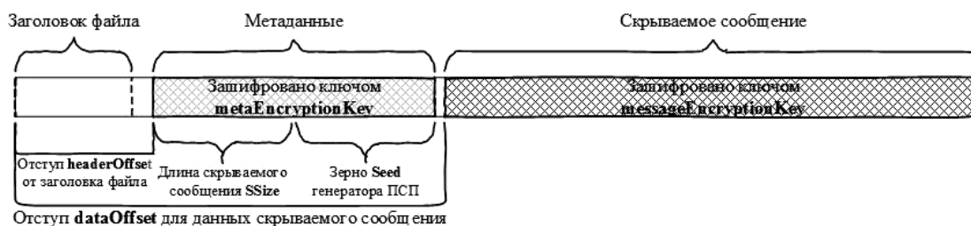
Рис. 2. Структура контейнера после записи секретного сообщения
