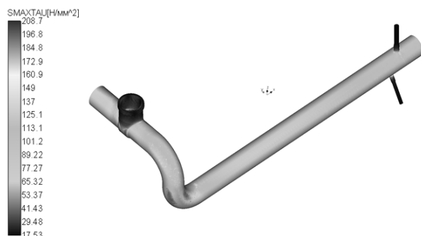
Рис. 4. Розподіл наведених напруг \sigma_{13} в ГЦТ («холодна» нитка, від ГЦН до КР; режим НЕ + МРЗ, навантаження – внутрішній тиск)
