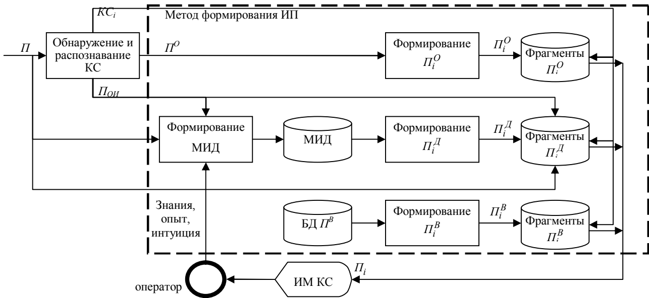
Рис. 1. Схема метода формирования ИП ИМ КС
