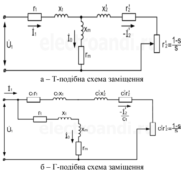
Рис. 1. Схеми заміщення асинхронного двигуна
