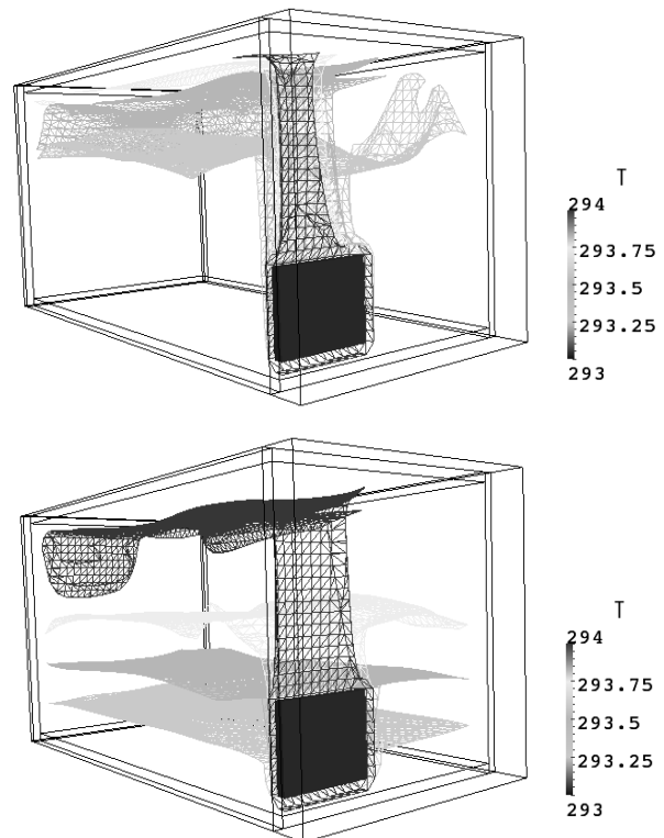
Рис. 1. Ізоповірки температури
