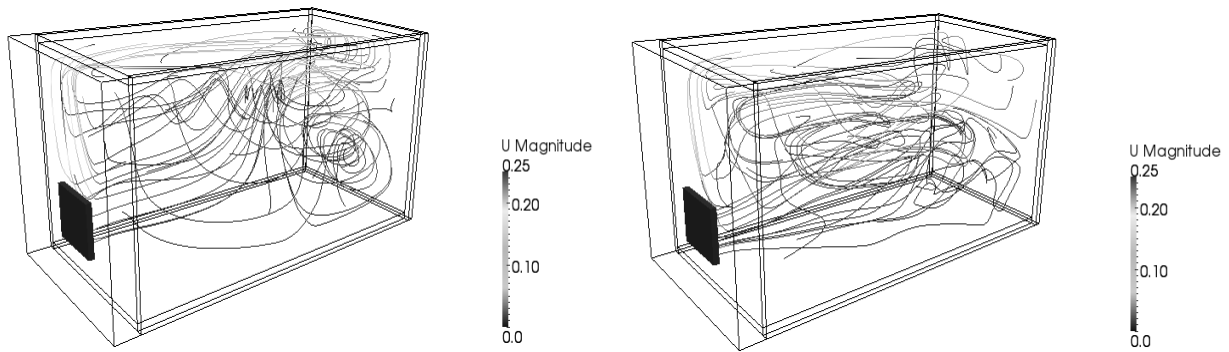
Рис. 2. Лінії струму
