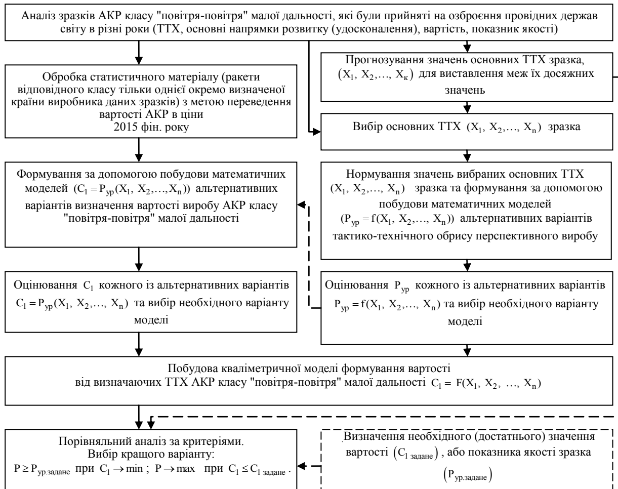
Рис. 1. Загальна схема методичного підходу обґрунтування тактико-техніко-економічного обрису авіаційної керованої ракети класу "повітря-повітря" малої дальності
