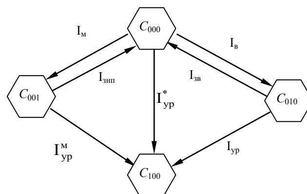
Рис. 1. Граф виконання завдання радіолокаційного забезпечення мобільним радіолокаційним комплексом
