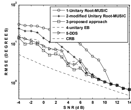
Рис. 1. СКО оценивания угловых координат ИШИ в зависимости от ОСШ
