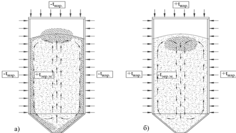
Рис. 1. Процесс теплообмена в силосе: а – при низкой температуре наружного воздуха; б – при высокой температуре наружного воздуха
