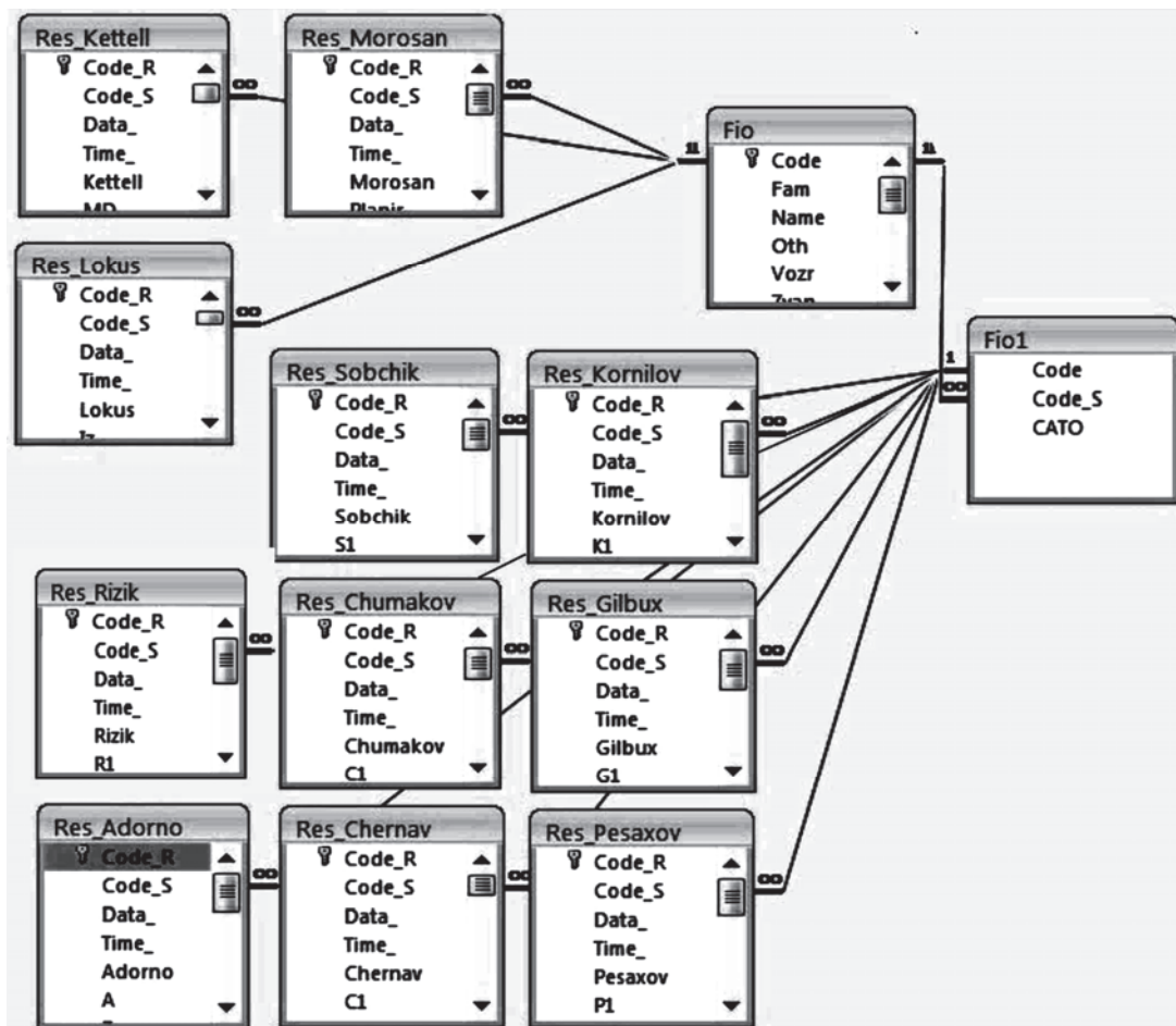
Рис. 1. Схема таблиць у БД та їх взаємозв'язок
