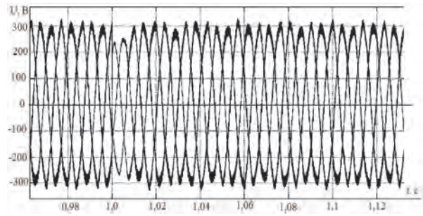
Рис. 3. Осциллограмма напряжения на статорной обмотке АСТГ при изменении нагрузки
