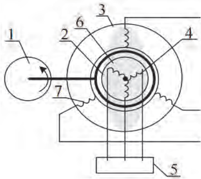
Рис. 1. Схема АСТГ
