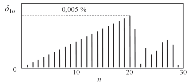
Рис. 3. Відносна похибка відтворення нормованого рівномірного спектра ( f_0 = 100 Гц)
