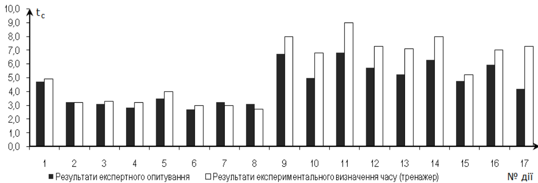
Рис. 6. Порівняльна характеристика результатів експертного опитування та експериментального визначення середнього часу необхідного для виконання дій авіаспеціалістом у випадку відмови двигуна на зльоті
