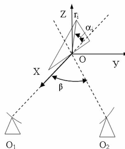
Рис. 1. Система координат
