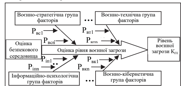
Рис. 3. Приклад декомпозиції загрози воєнній безпеці держави з використанням методу Ісакаві
