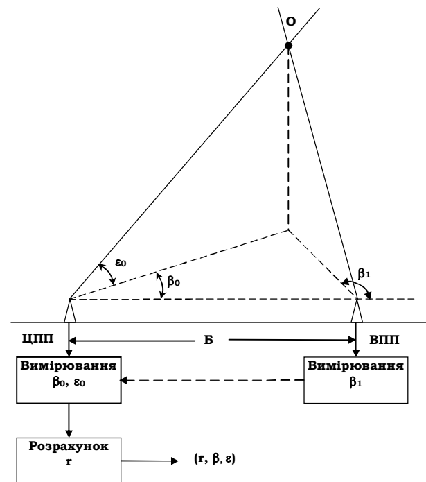
Рис. 1. Узагальнена структурна схема системи пасивної локації з кутомірним методом вимірю координат
