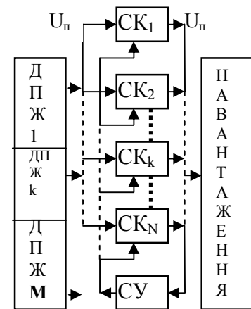
Рис. 1. Структура модульного ППН
