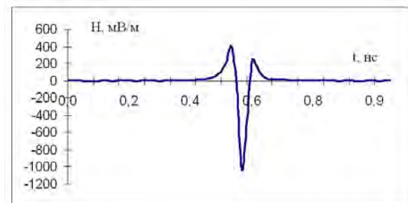
Рис. 4. Форма НШС сигналу у напрямі головного максимуму
