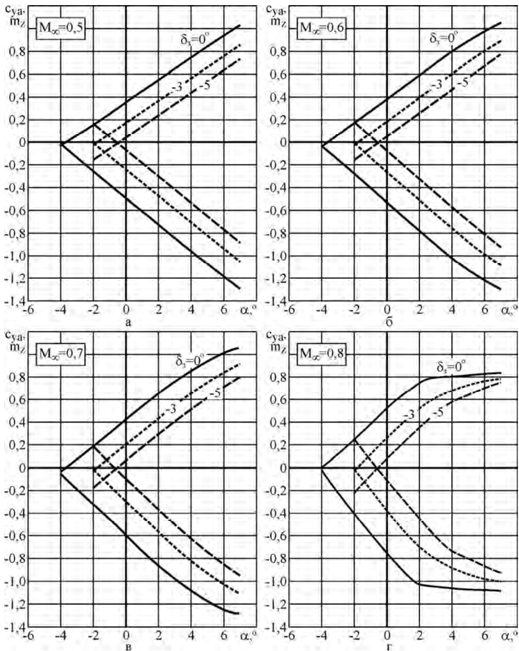
Рис. 3. Зависимости коэффициента подъемной силы и коэффициента продольного момента от угла атаки: а – M_\infty = 0,5 ; б – M_\infty = 0,6 ; в – M_\infty = 0,7 ; г – M_\infty = 0,8
