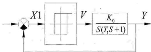
Рис. 1. Структурна схема моделювання нелінійності
