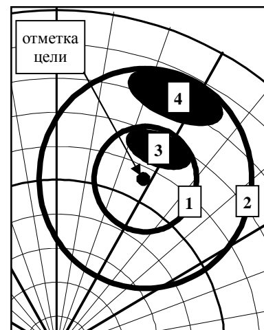
Рис. 3. Форма стробов при обычной (стробы 1 и 2) и подпороговой (стробы 3 и 4) обработке
