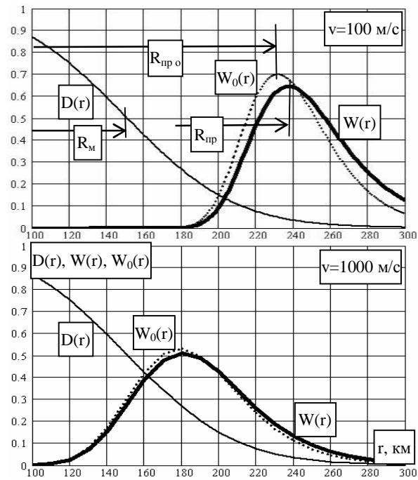
Рис. 1. Зависимость вероятности обнаружения D(r) , плотностей вероятности W(r) и W_0(r) от дальности r
