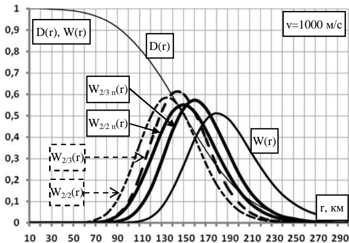
Рис. 2. Зависимость вероятности D(r) , плотностей вероятности W_{2/2}(r), W_{2/3}(r), W_{2/2п}(r), W_{2/3п}(r) от дальности r для скоростной приближающейся цели
