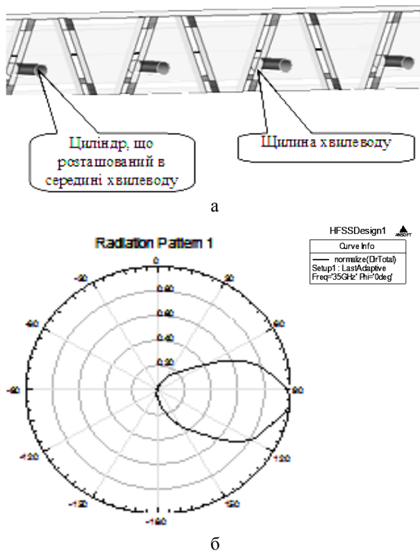
Рис. 5 Хвилеводно-щілинна антенна ПРД системи «Вітим» в HFSS v. 13.0 зі зміненою конструкцією (циліндри в середині хвилеводу): а – зовнішній вигляд; б – діаграма спрямованості
