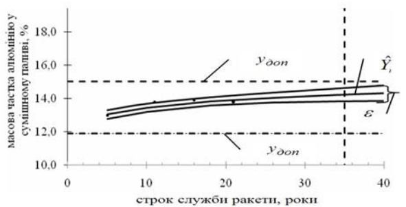
Рис. 8. Прогнозування значення масової частки алюмінію у паливі двигунів РДГТ-295
