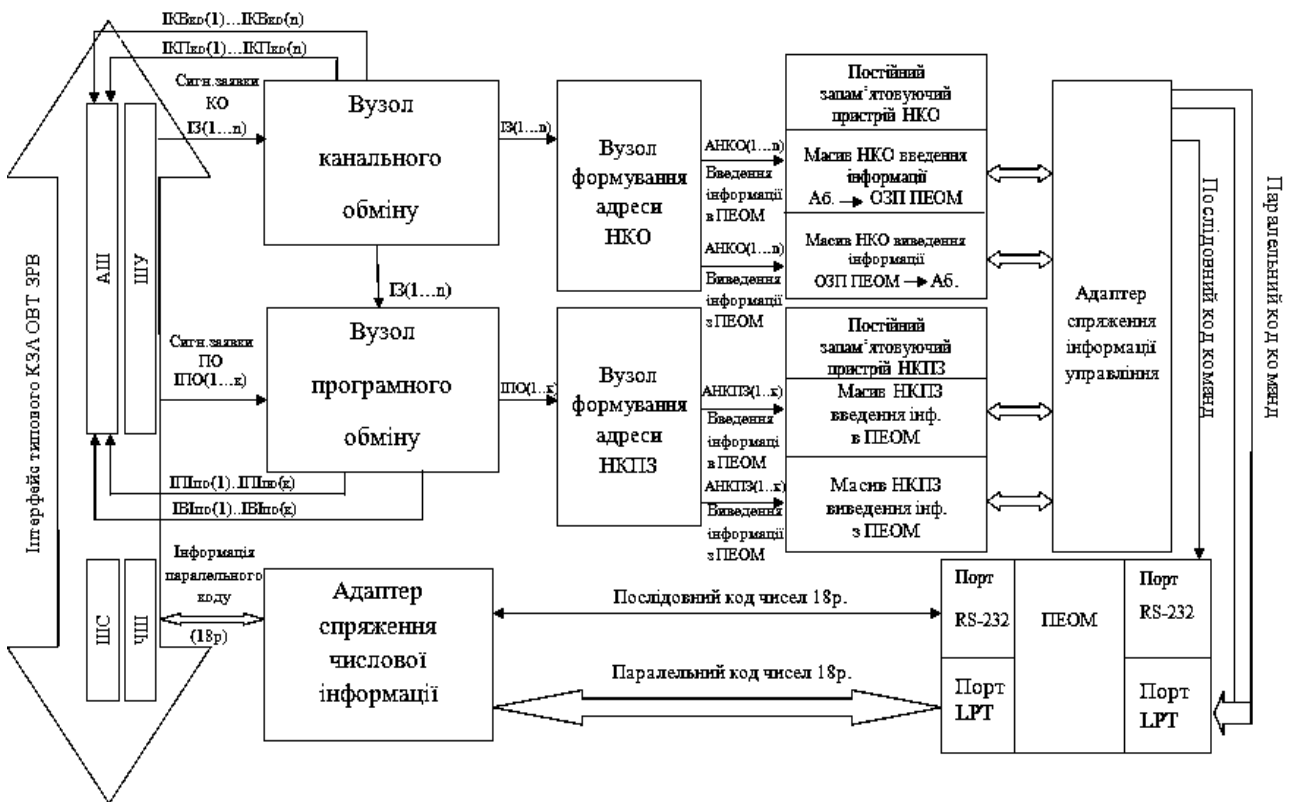
Рис. 1. Структурна схема пристрою інформаційного спряження ПЕОМ та типового інтерфейсу КЗА ОБТ ЗРВ
