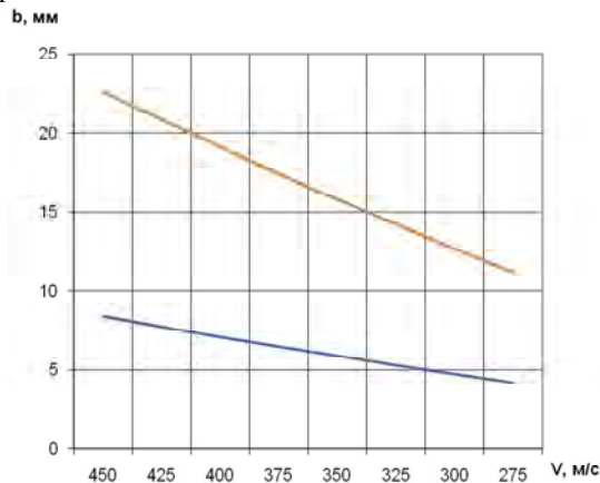
Рис. 4. Залежність пробиття сталеві перешкоди від швидкості кулі
