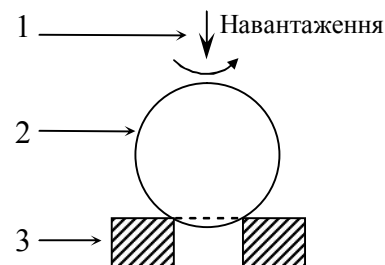
Рис. 1. Схема випробування: 1 – напрямок навантаження; 2 – рухомий зразок; 3 – нерухомий зразок
