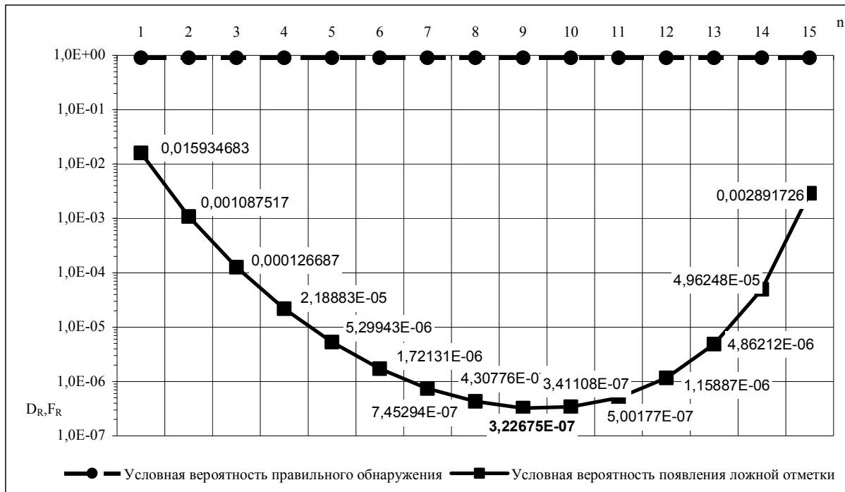
Рис. 2. Залежність характеристик виявлення від числа суммуємих кадрів
