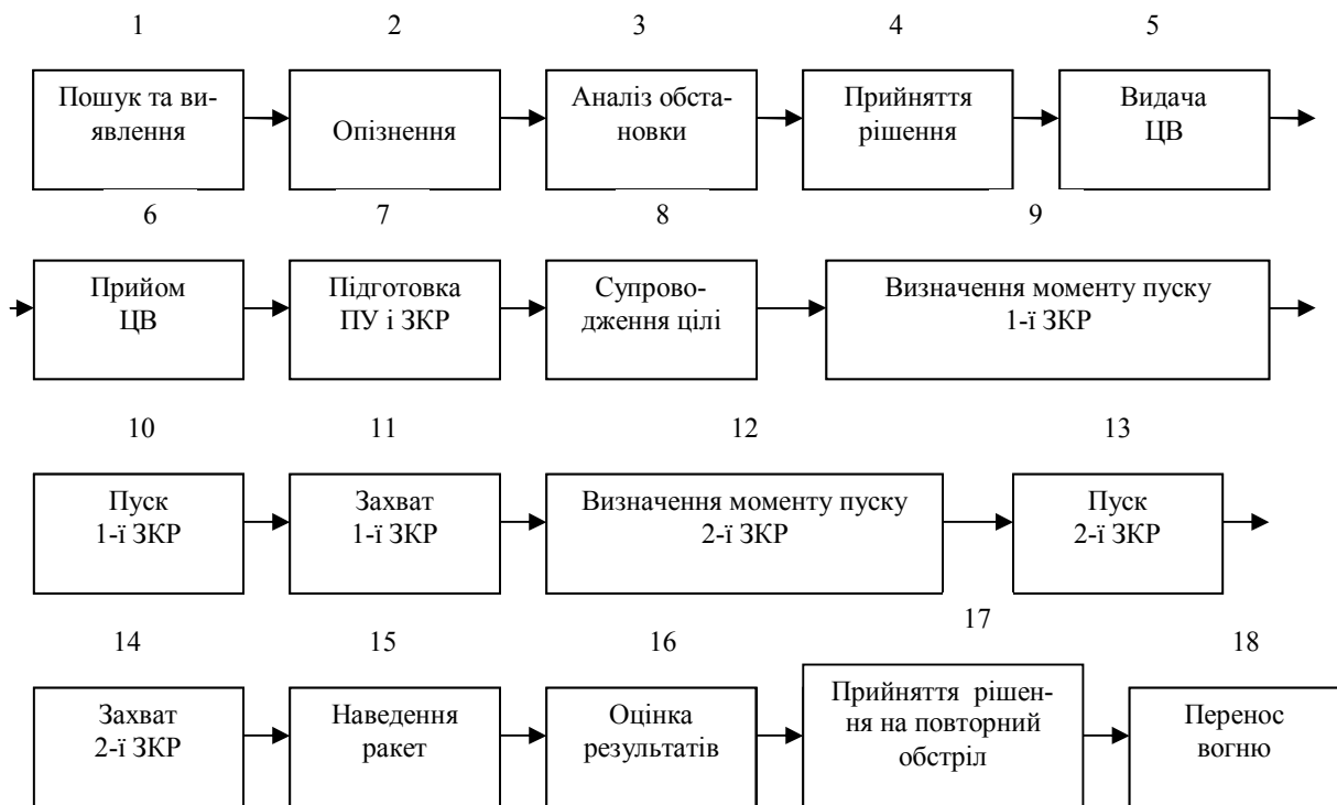
Рис. 1. Алгоритм бойової роботи ЗРК «Оса-МА»
