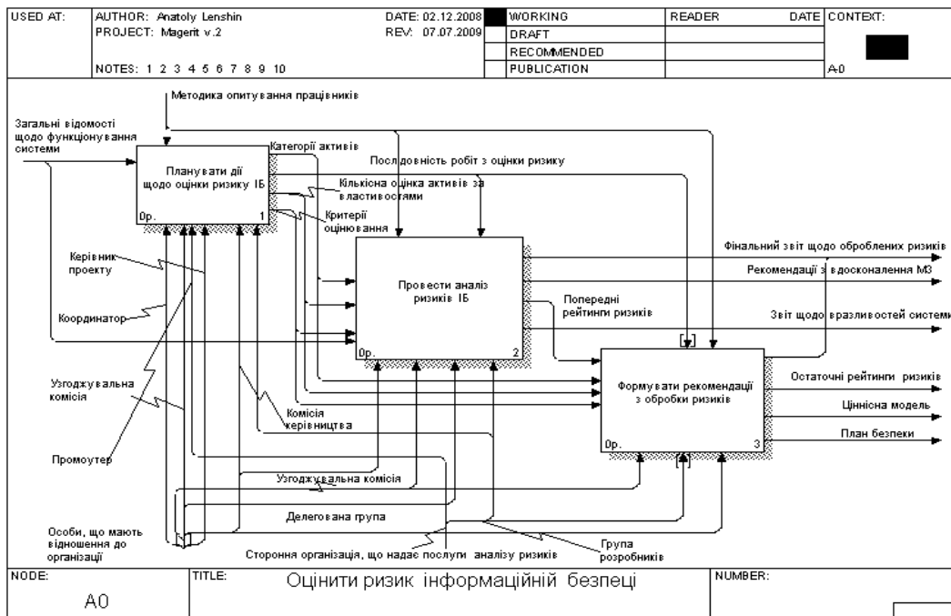
Рис. 3. Декомпозиція метапроцесу ОР у нотатції IDEF-0
