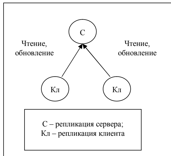
Рис.1. Стратегия репликации клиент-сервер
