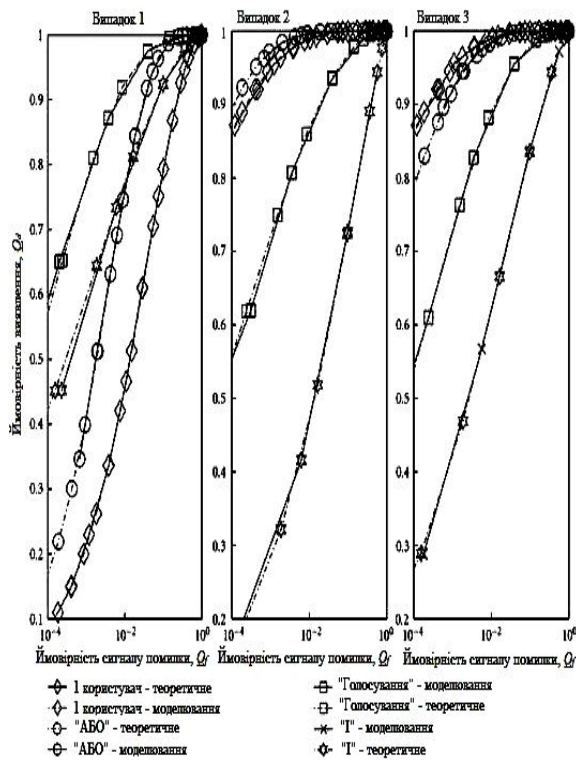
Рис. 8. ROC для 5 взаємодіючих користувачів в каналі з AWGN в 3 випадках:
