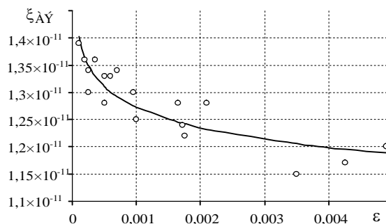
Рис. 7. Зависимость удельной эмиссионной активности \xi_{AЭ} от износа \varepsilon
