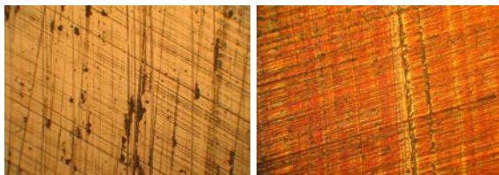
Рис. 6. Фрактография поверхностей трения трибосистемы с ионно-плазменными покрытиями, работающими в условиях наноизнашивания \times 450 : а – MoN; б – TiAlN
