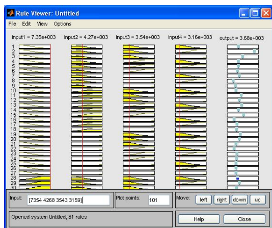
Рис. 4. Інтерфейс вікна генерованих правил системи ANFIS
