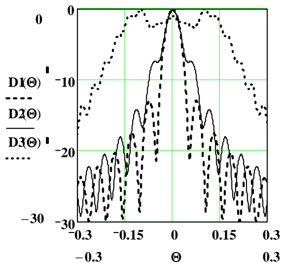
Рис. 2 Скалярне поле дифракції приймальної антени радіовибухувача
