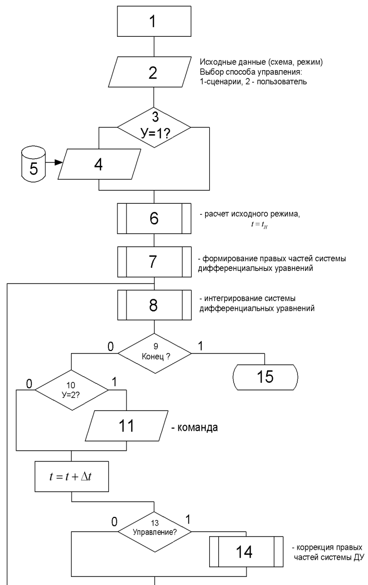
Рис. 1. Алгоритм программы имитационного моделирования
