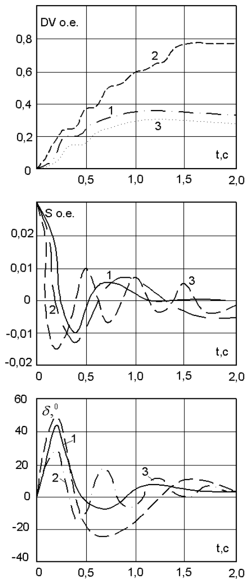
Рис. 2. Динамическое воздействие при DV, изменения скольжения s , угла ротора \delta при включении генератора типа ТВВ-200-2 в сеть методом самосинхронизации при \delta = 0^\circ , s = 0,02 , T_j (1 – схема по ЧХ; 2 – один контур «Электросила»; 3 – один контур И.М. Постников)
