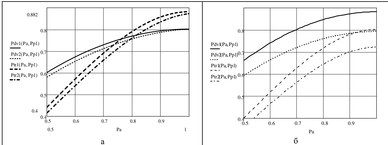
Рис. 1. Графічні залежності ІБР двоканального і триканального ПУ ЦТС від змінення ІБР АЗ при вихідних даних: а – P_{p1} = 0.9 , P_{ckd} = 0.99 , P_{me} = 0.99 , P_{vs} = 0.99 ; б – P_{p1} = 0.99 , P_{ckd} = 0.9 , P_{me} = 0.9 , P_{vs} = 0.9
