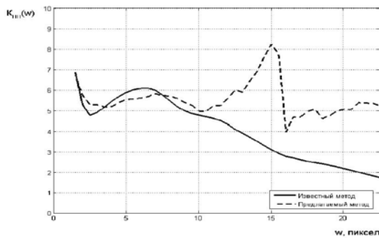
Рис. 5. Зависимость коэффициента подавления помехи K_{\text{п}}(w) от полуширины окна обработки
