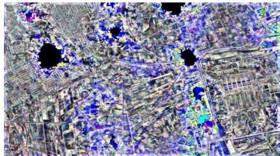
Рис. 4. Восстановленное изображение
