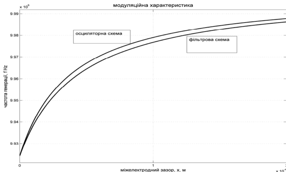
Рис. 2. Модуляційні характеристики КГ з модуляцією міжелектродного зазору
