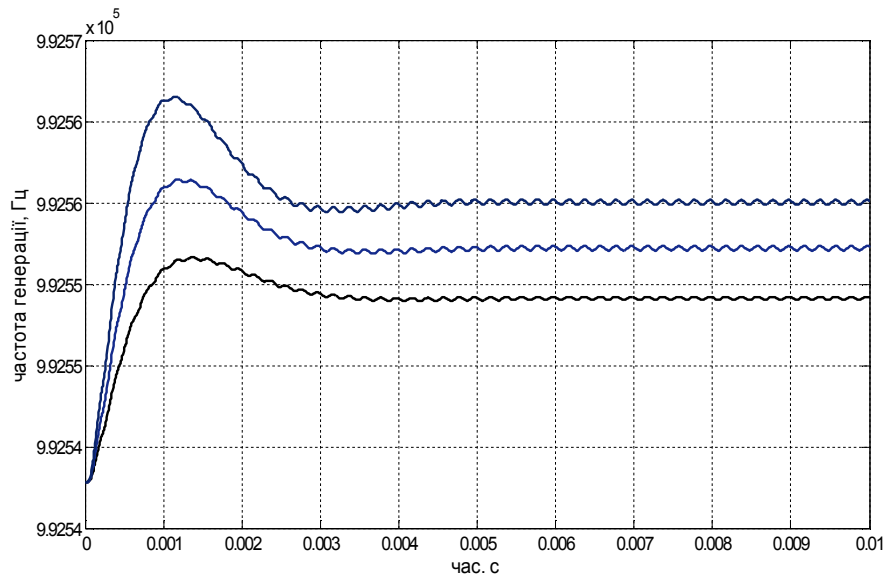
Рис. 8. Часова характеристика встановлення частоти КГ для різних значень шпаруватості імпульсів збудження ЛІДП
