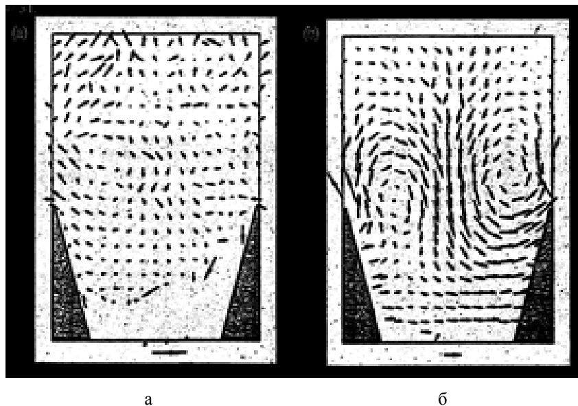
Рис. 1. Вторинні вихрові структури в околі оребреної поверхні [8 – 10]: а – s^+ = 15 ; б – s^+ = 31
