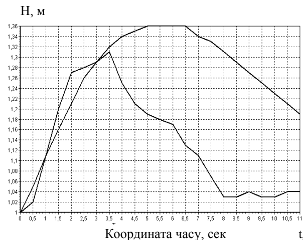
Рис. 5. Залежність відносної частоти обертання та величини напору турбіни від часу
