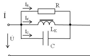
Рис. 1. Параллельное включение R, L к , C
