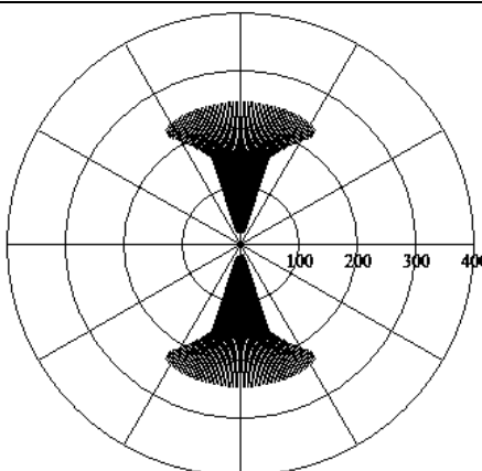
Рис. 7. Розрахункова зона виявлення цілей з ЕВП 1 м 2 літаком ДРЛВіУ типу "Хокай-2000" над морем
